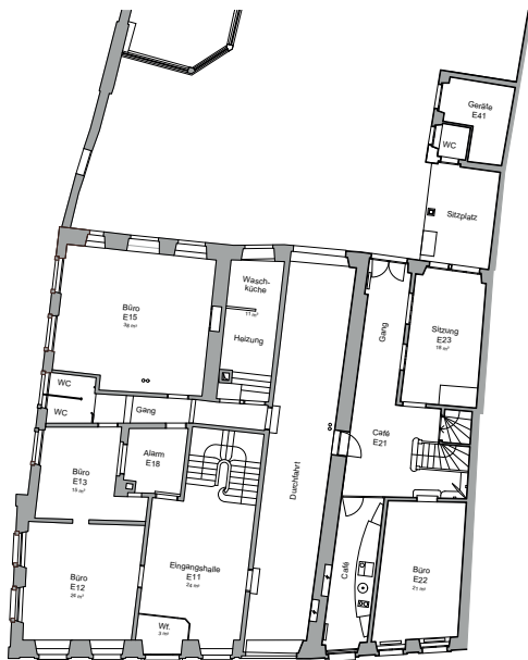
Erdgeschoss Hauptgebäude
