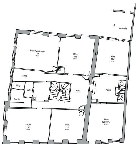
1. Obergeschoss
