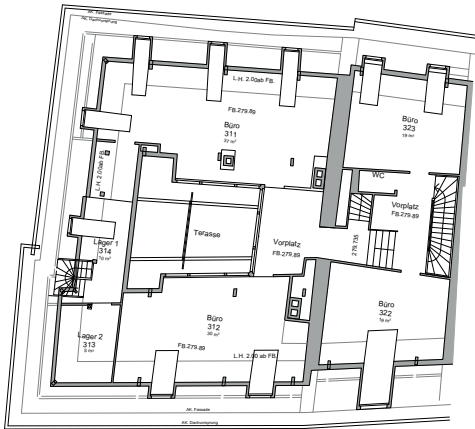
3. Obergeschoss
